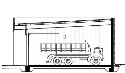
SCHNITT A-A / SEZIONE A-A
