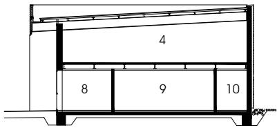
SCHNITT B-B / SEZIONE B-B
