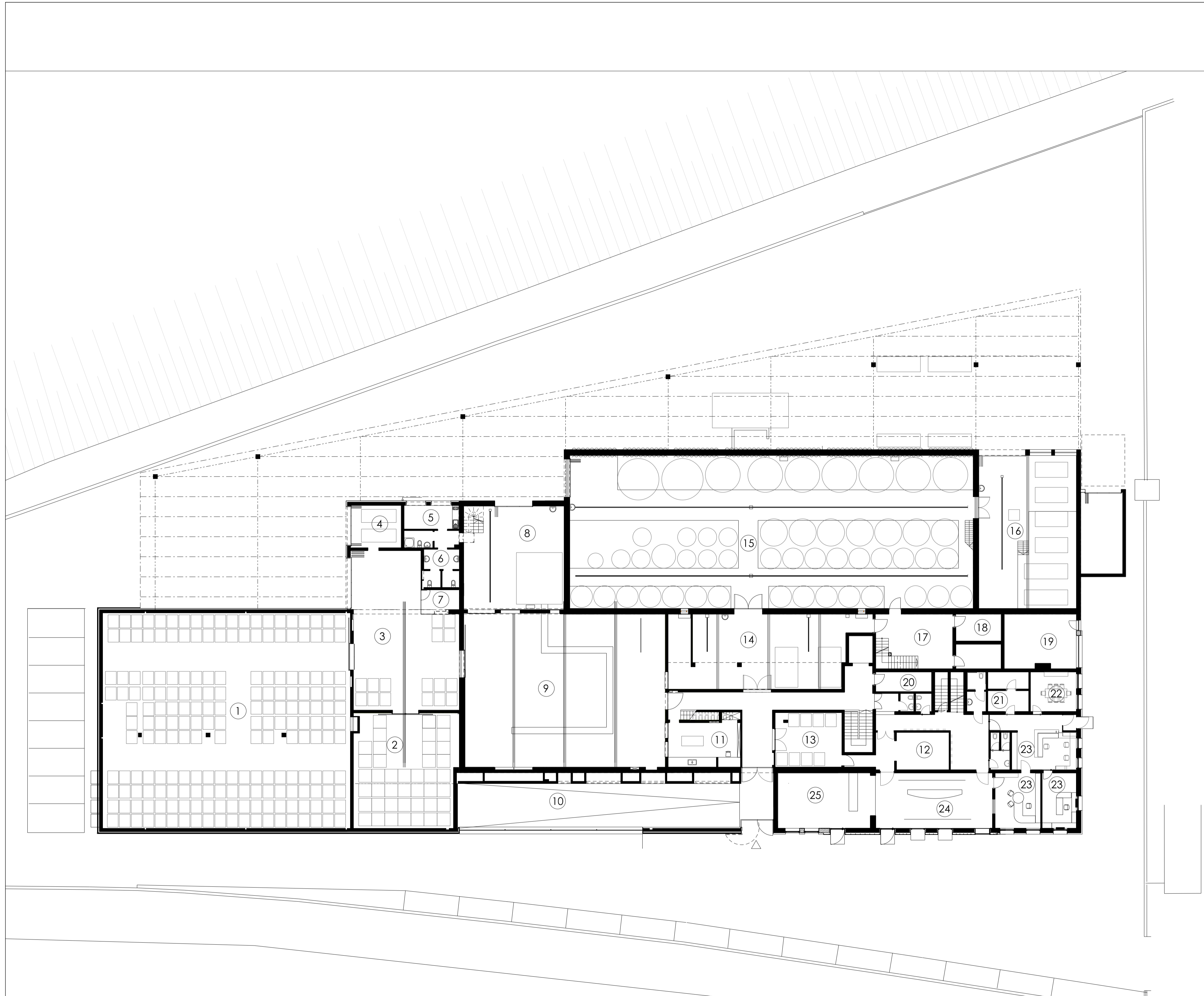
Eisacktaler Kellerei (Klausen) / Cantina valle Isarco (Chiusa) - Grundriss Erdgeschoss - Pianta piano terra
