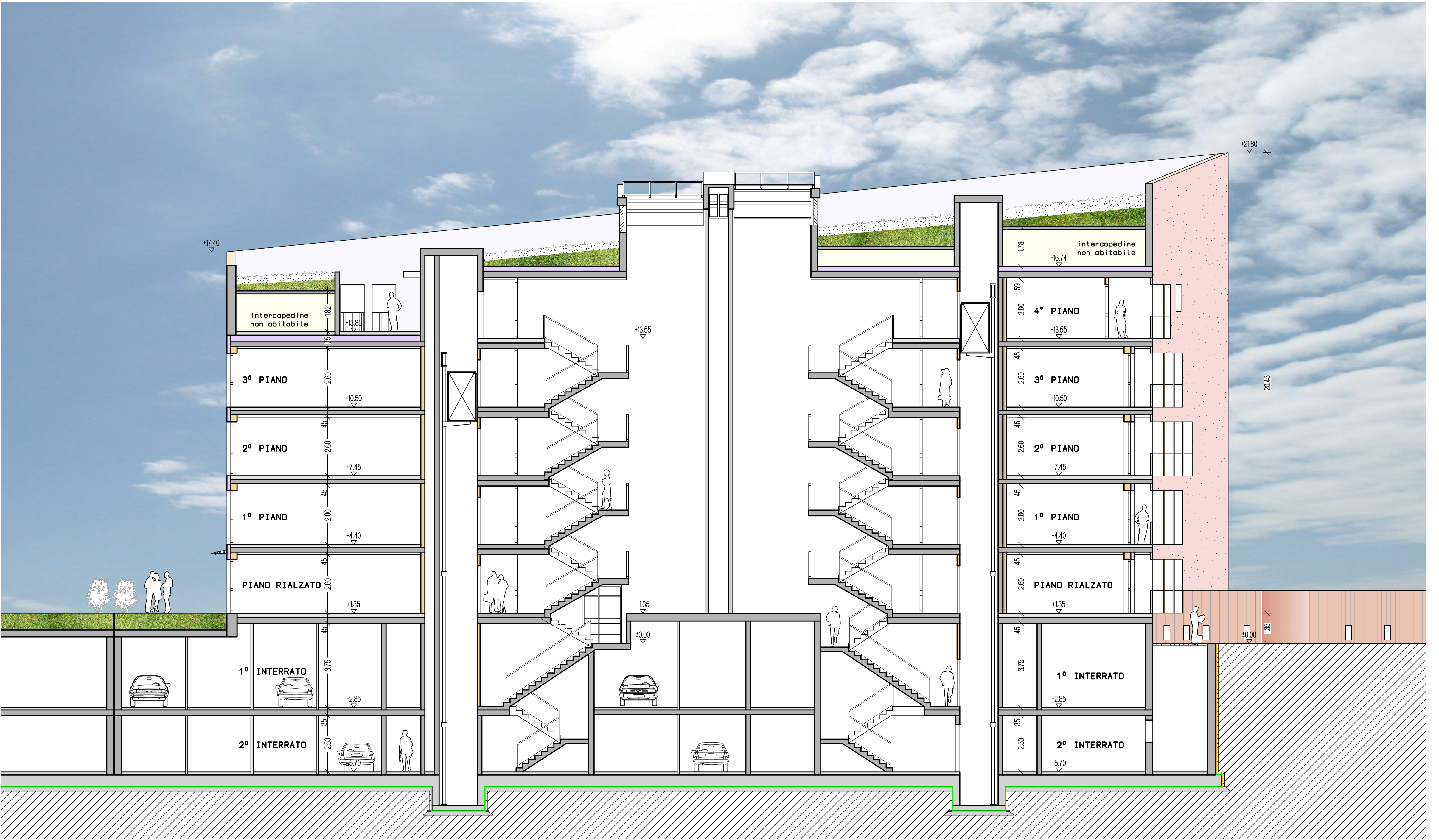
SEZIONE 2-2
