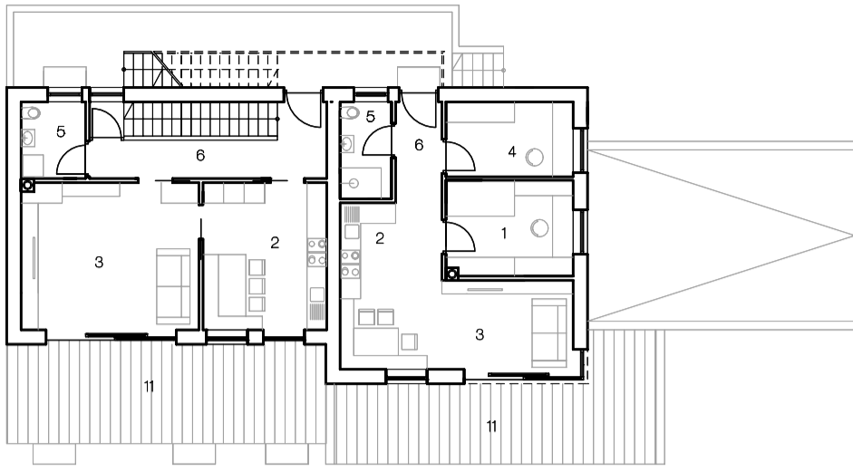
ERDGESCHOSS
