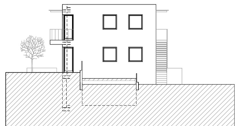
OSTANSICHT
