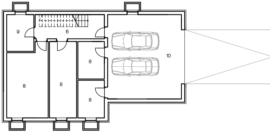
KELLERGESCHOSS
