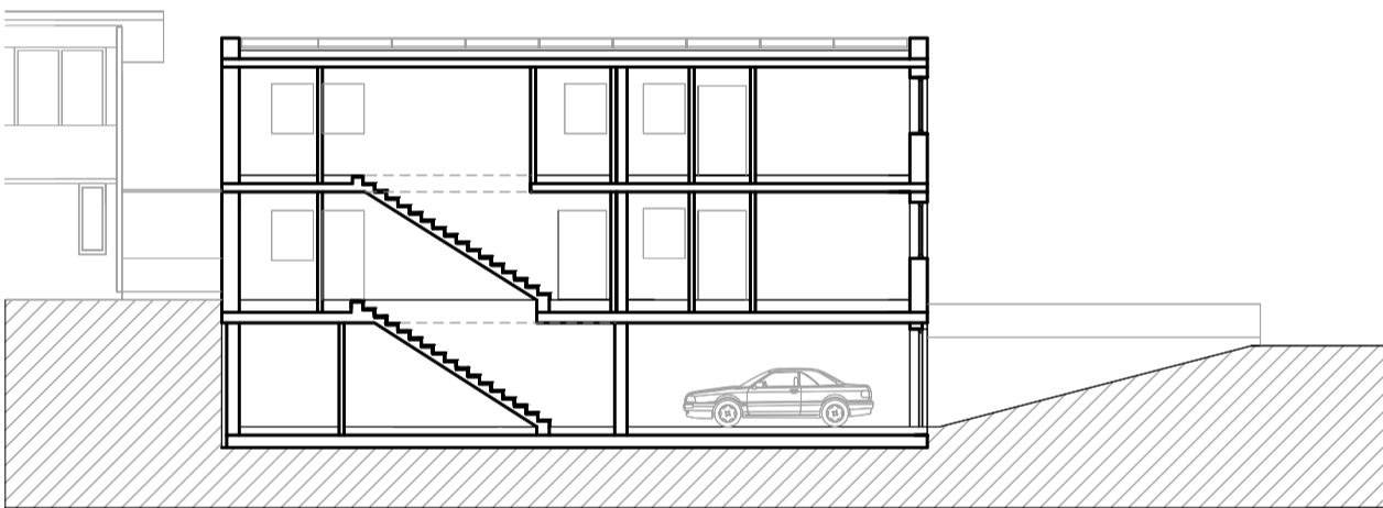
SCHNITT AA
