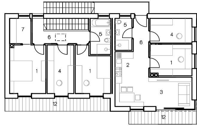
OBERGESCHOSS
