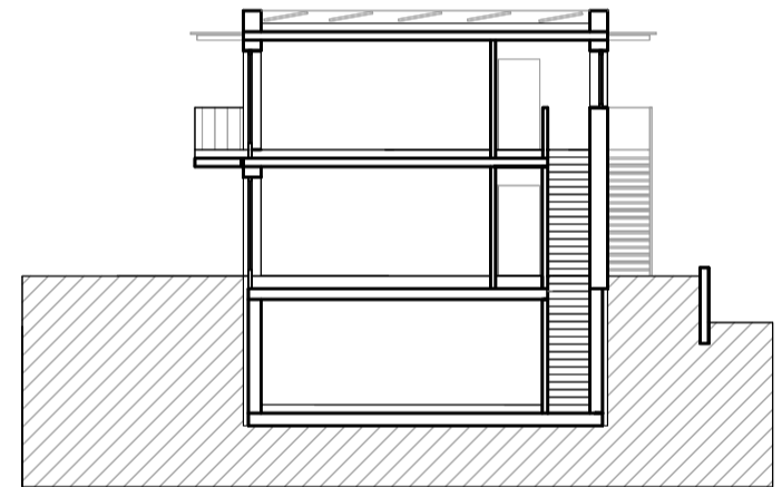
SCHNITT BB
